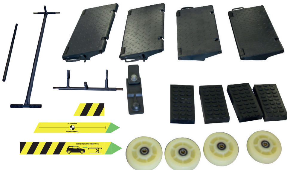
Ausgepackte Kleinteile; Auffahrampen (4 Stk.), Fahrwerks-Verbindungsstück (1), Fahrwerksrollen (4 Stk.) und Sicherheitssticker (6 Stk.)
