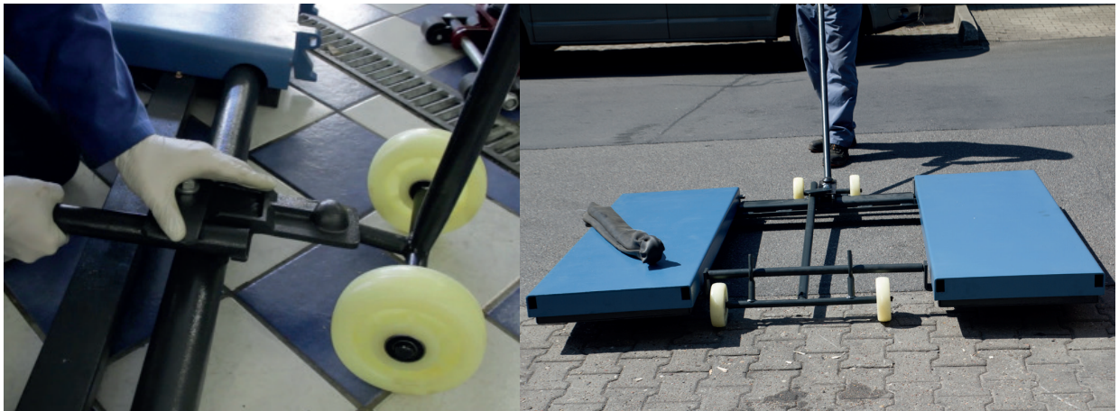
Sichern des unteren Fahrwerks !
