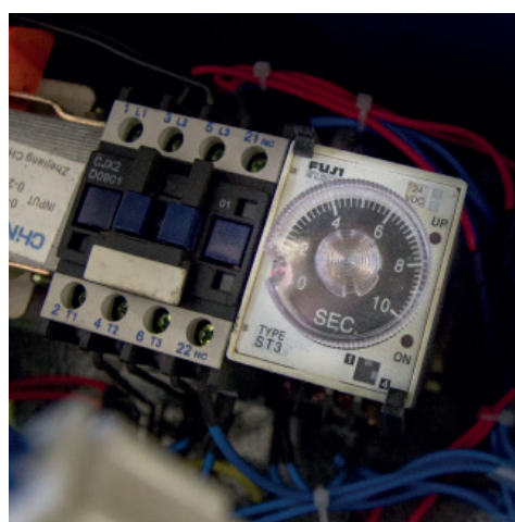
geöffnetes Bedienpult mit Zeitschaltuhr (in weiß). Abb.25.27
