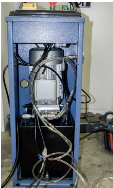
Ansicht einer korrekten Verkabelung zum Bedienpult:
