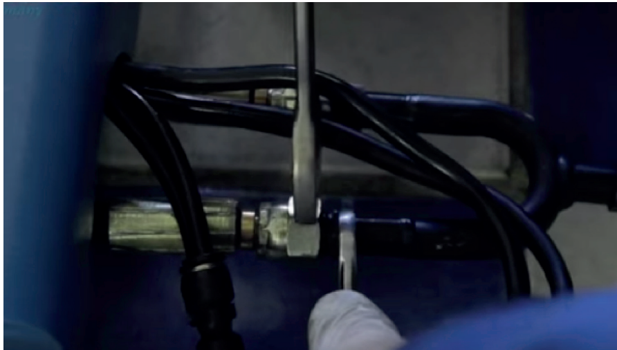
Anschrauben des Y-Stückes innerhalb des Bedienpults
