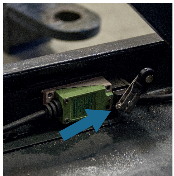
Klemmschraube lösen Rollentaste einstellen Abb.28.1
