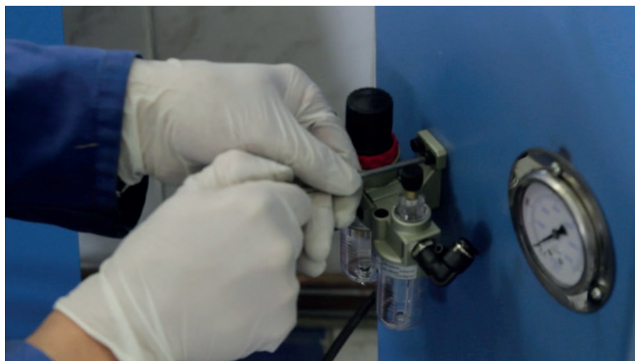
Anschrauben des Druckminderers.
